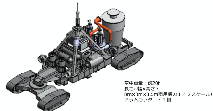
採鉱試験機イメージ
